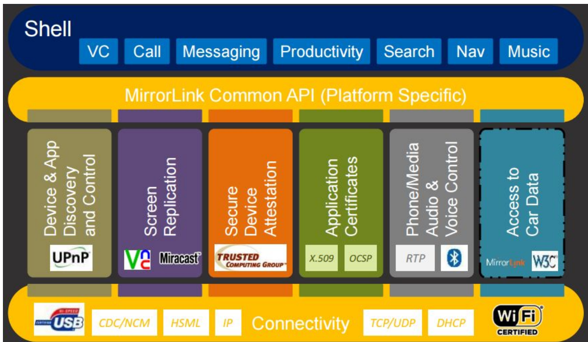
Figura 3.9. Arquitectura Mirrorlink.
