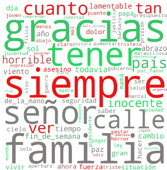
Figura 30: Análisis de polaridad para la reacción SAD.
