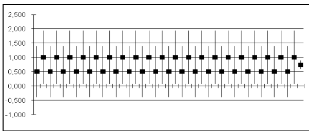
Figura 8: Diagrama de árbol que resultan de agregar los experimentos: E1 a E20 con : media 1 = 100, media 2 = 90, desvío std 1 = 10, desvío std 2 = 9, y E21 a E40 con: media 1 = 100, media 2 = 95, desvío std 1 = 10, desvío std 2 = 9, incluyendo 25 sujetos experimentales por brazo por cada experimento.
