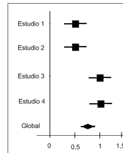
Figura 6: Diagrama de árbol que resultan de agregar los experimentos: E1, E2 con: media 1 = 100, media 2 = 90, desvío std 1 = 10, desvío std 2 = 9, y E3, E4 con: media 1 = 100, media 2 = 95, desvío std 1 = 10, desvío std 2 = 9, incluyendo 100 sujetos experimentales por brazo por cada experimento.
