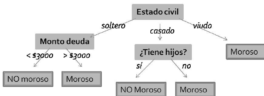
Fig. 46. Árbol de decisión
