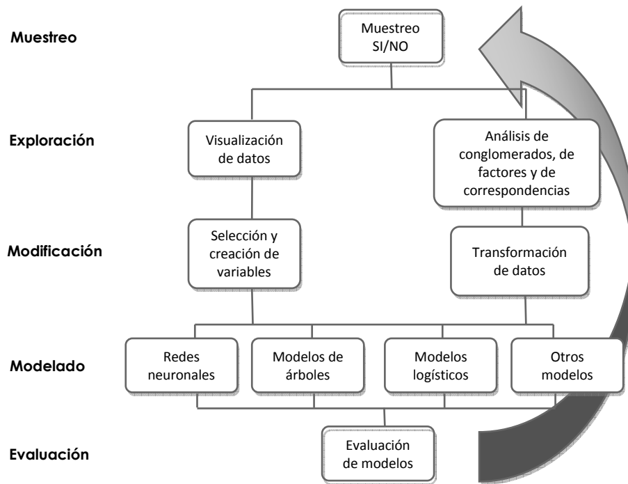
Fig. 5. Iteración de fases en SEMMA
