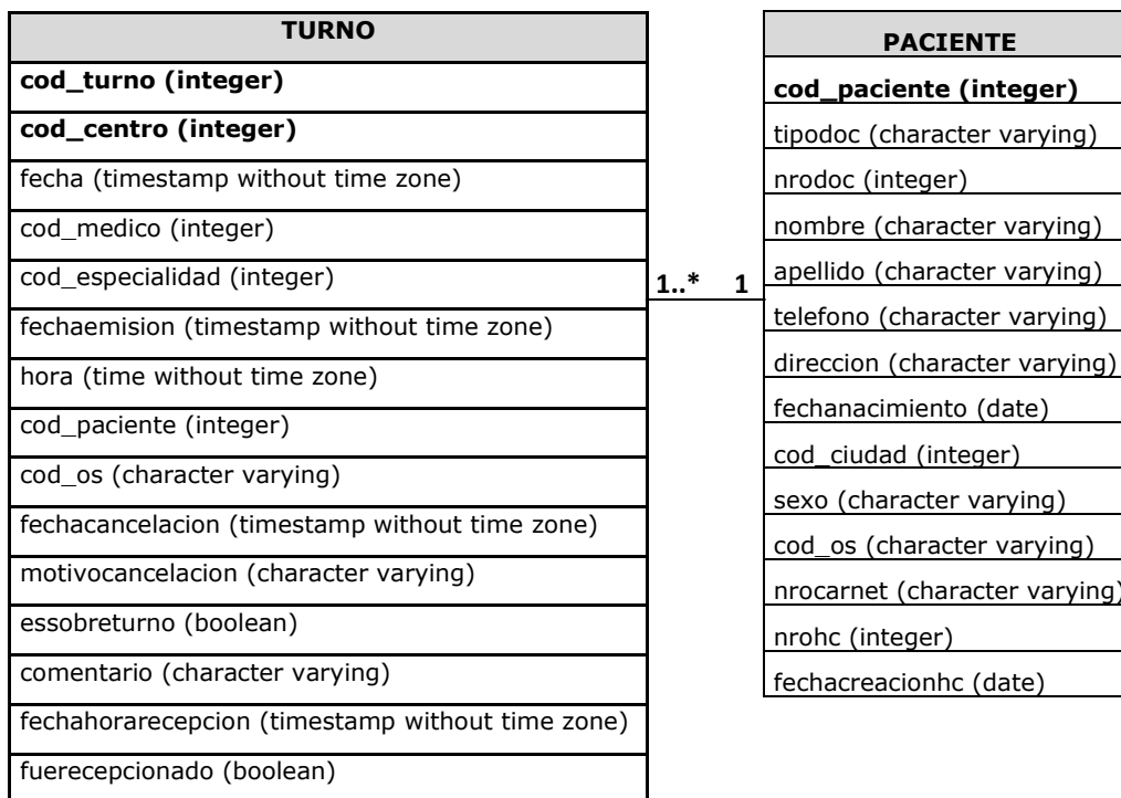
Fig. 14. Estructura de las tablas Turno y Paciente
