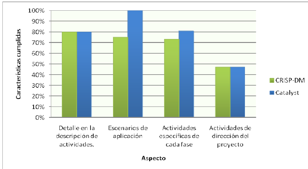
Fig. 45. Porcentaje de características presentes en cada metodología
