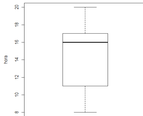
Fig. 21. Distribución de la variable hora.
