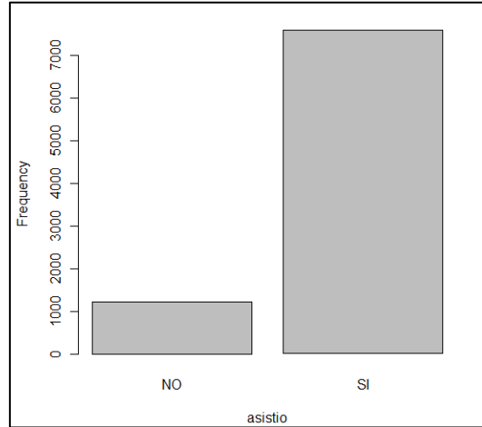
Fig. 30. Distribución de la variable explicada
