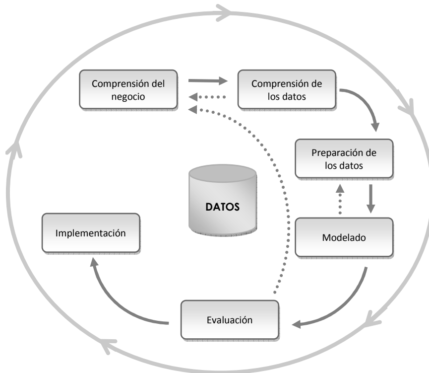
Fig. 6. Metodología CRISP-DM
