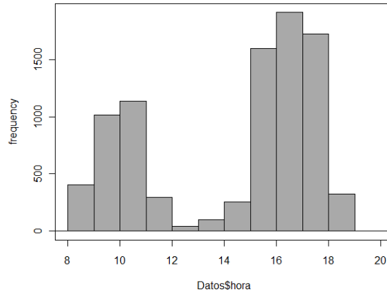
Fig. 22. Histograma de la variable hora.
