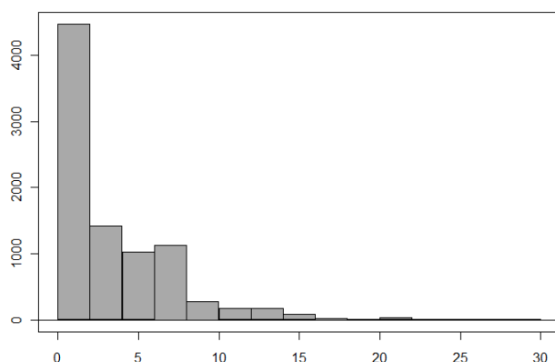
Fig. 23. Histograma de la variable "días antelación solicitud"
