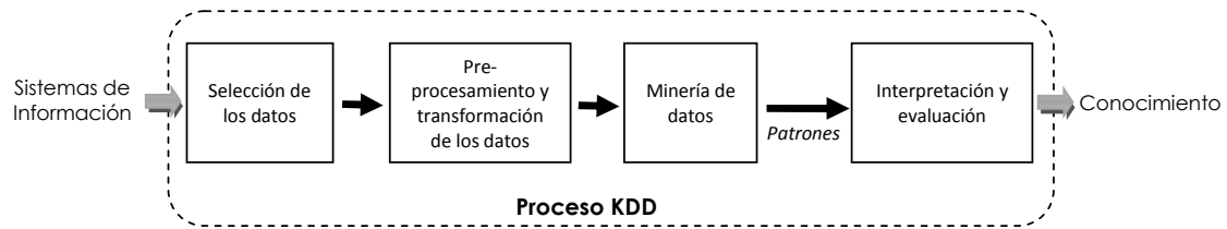
Fig. 3. Esquema del proceso KDD resumido
