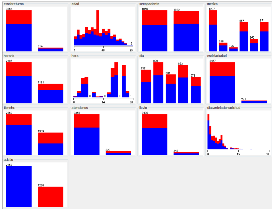
Fig. 37. Distribución del conjunto de datos muestreado.
