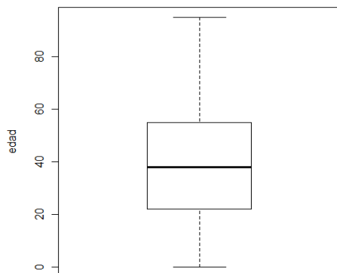
Fig. 20. Distribución de la variable edad.
