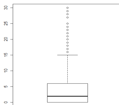
Fig. 24. Diagrama de cajas de la variable "días antelación solicitud"
