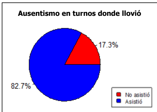
Fig. 27. Tasa de ausentismo cuando llovió.
