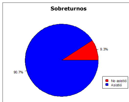
Fig.17. Tasa de ausentismo para los sobretornos
