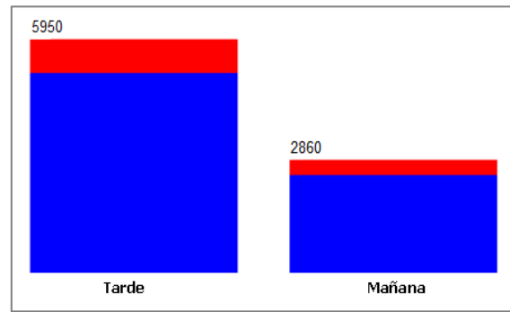
Fig. 26. Distribución de la nueva variable "horario".
