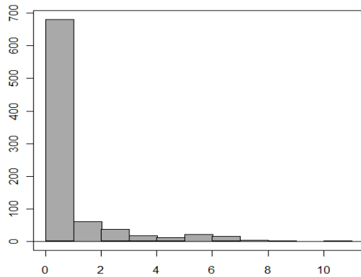
Fig. 25. Distribución de la variable "días antelación solicitud" en los sobretornos.
