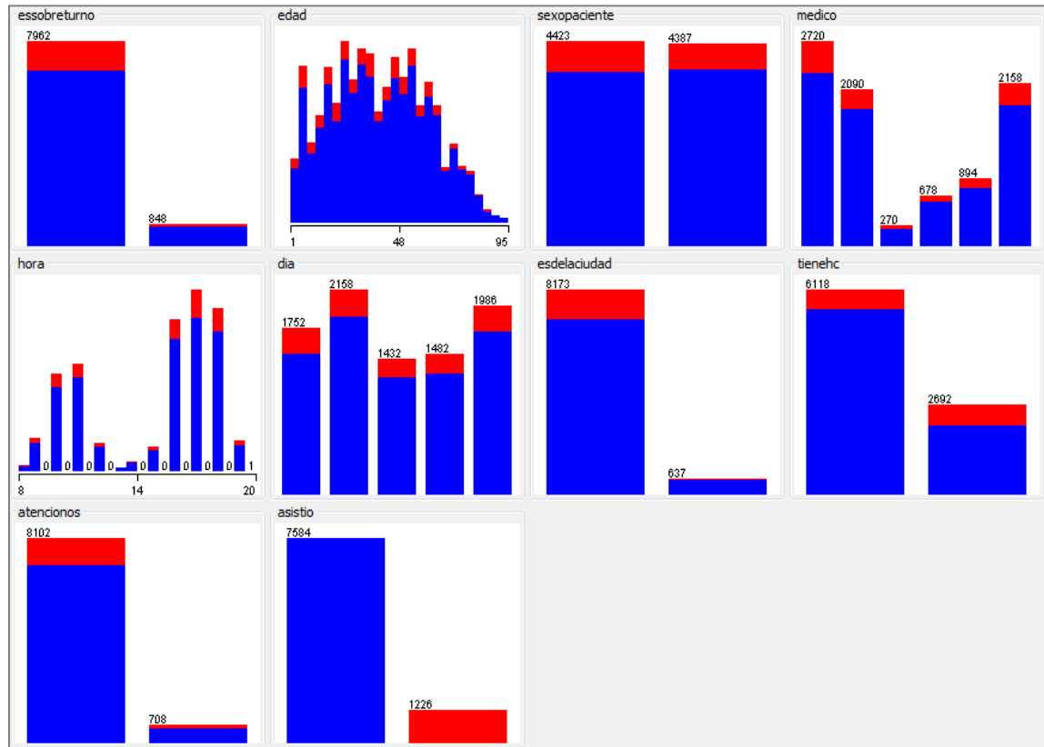
Fig. 16. Distribución de las variables del conjunto de datos.
